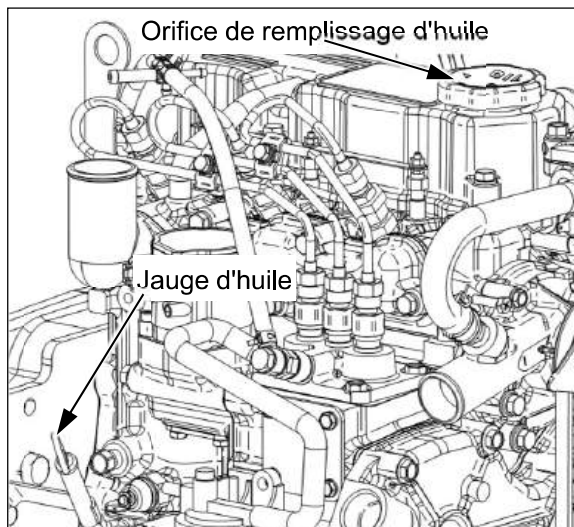
Jauge d'huile moteur
